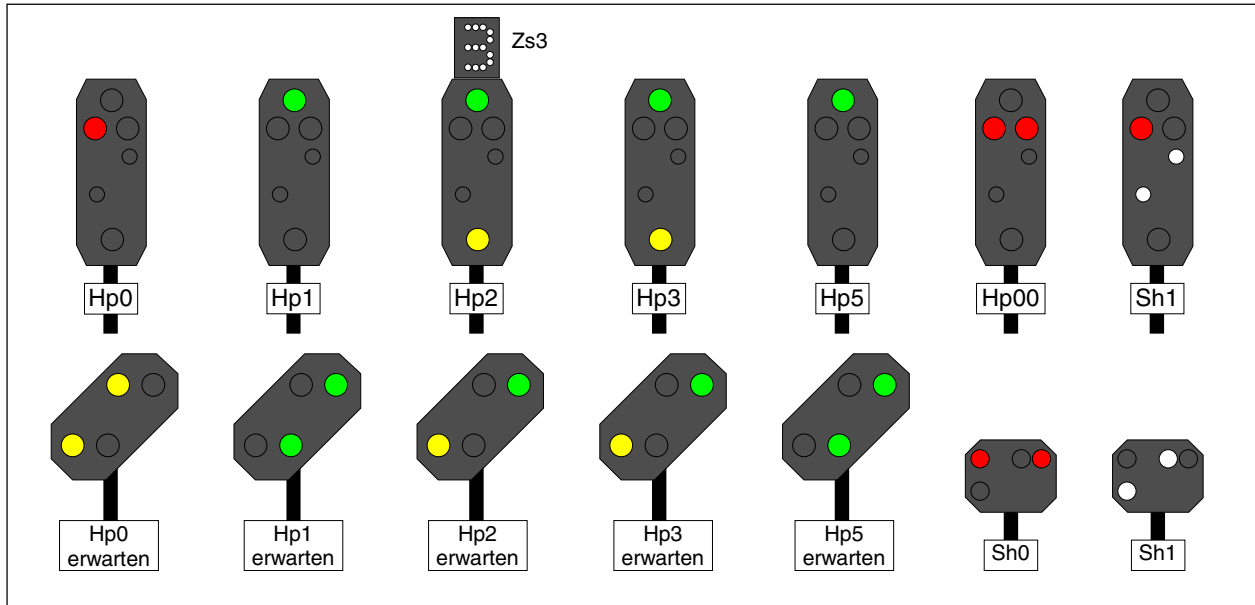
Abbildung 72: Signalbilder für Landeskennung D (DB Deutsche Bahn) und Zs3 < 40 km/h
