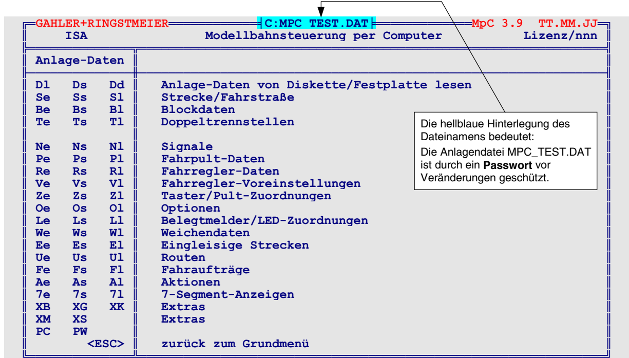
Abbildung 9: Bildschirmaufbau im Programmteil "Anlage-Daten"
