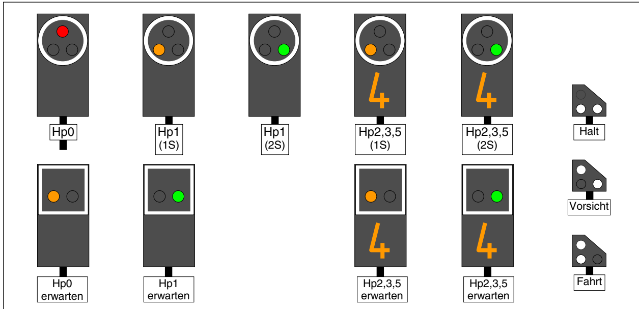
Abbildung 76: Signalbilder für Landeskennung C (SBB Schweiz, 'System N')
