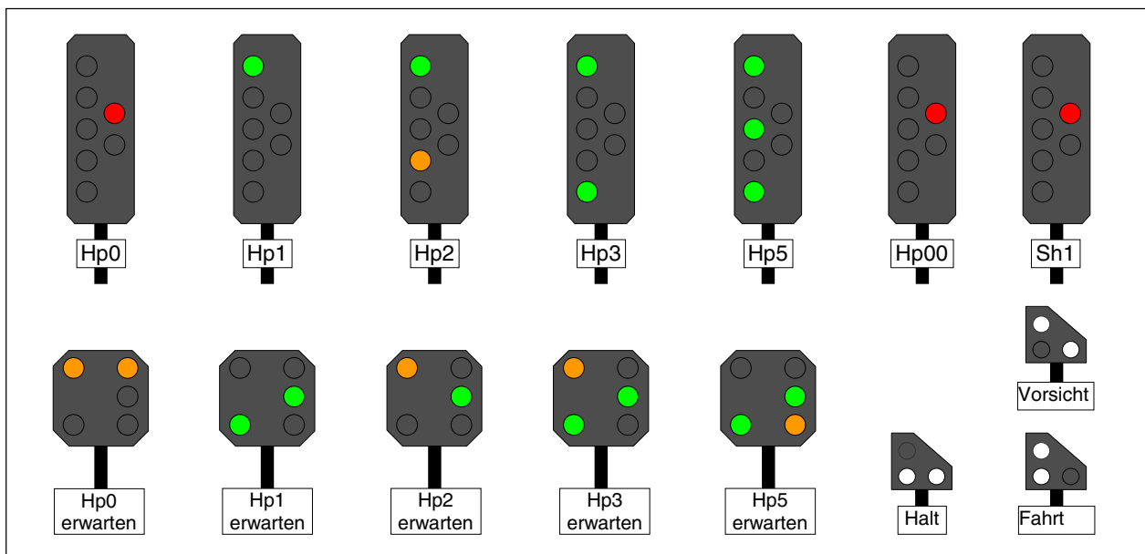
Abbildung 77: Signalbilder für Landeskennungen H und W (SBB Schweiz, 'System L')
